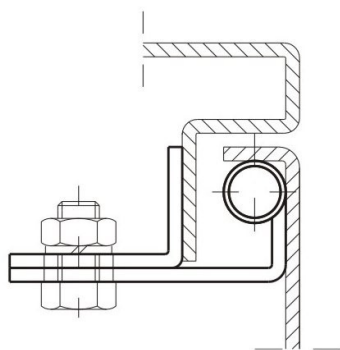
RT12P Cat.No. 03.175
