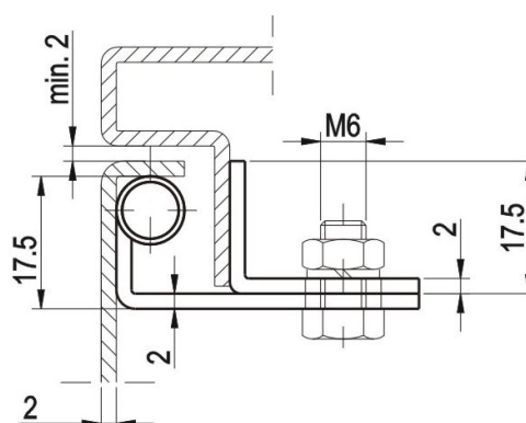
RT12L Cat.No. 03.176
