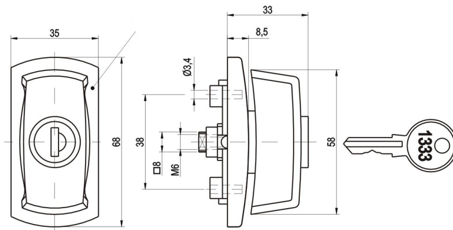
RW200/M Cat.No. 03.077
