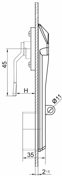
Lock Z40 Cat.No. 03.1060
