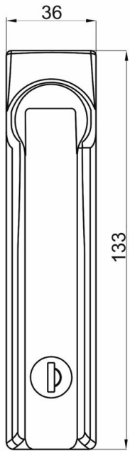
Lock Z39 Cat.No. 03.1058
