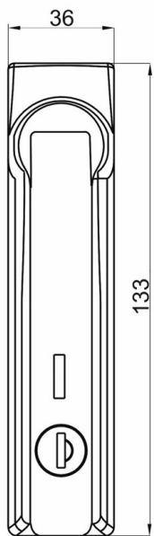
Lock Z40 Cat.No. 03.1060
