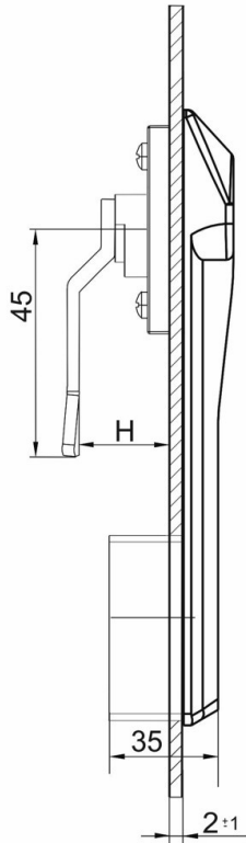
Lock Z39 Cat.No. 03.1058
