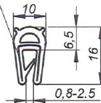
Ocelová vložka
