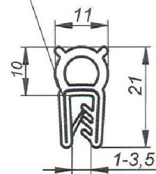
Ocelová vložka
