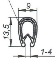
Ocelová vložka
