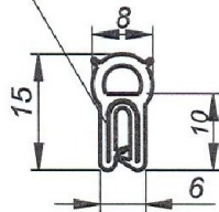
Ocelová vložka
