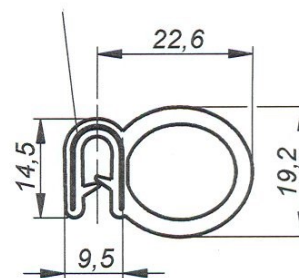
Ocelová vložka
