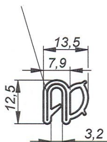
Ocelová vložka
