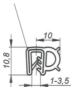
Ocelová vložka
