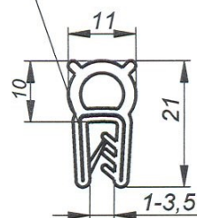
Ocelová vložka
